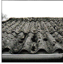
Welleternit und Wellbitumenplatten
